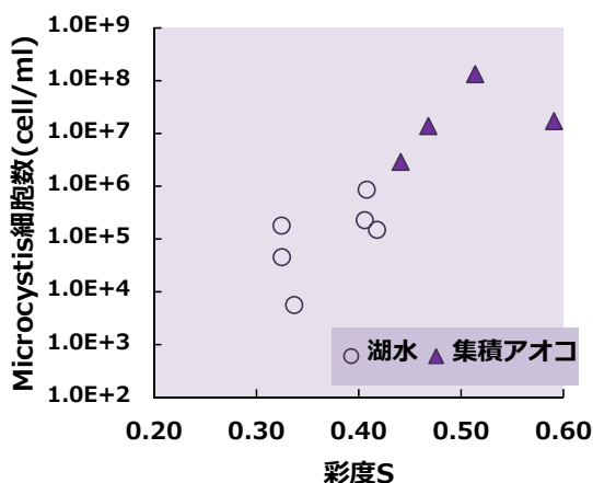
図1 彩度とMicrocystis細胞数の関係
