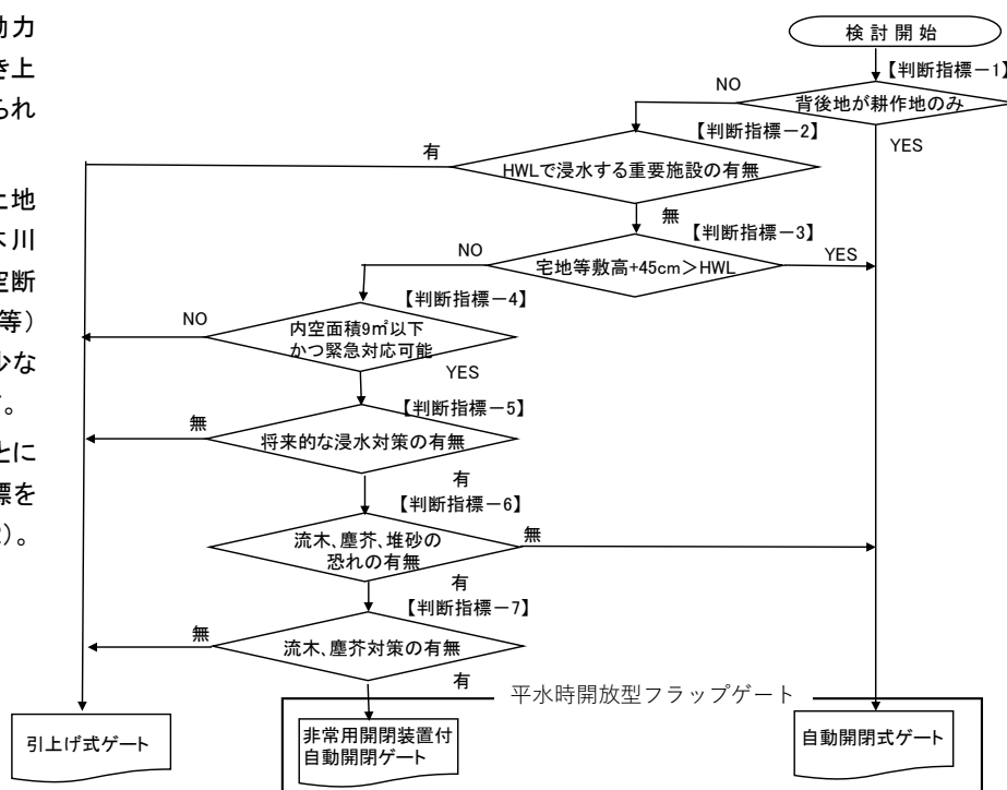
図2 無動力化判断指標作成例
