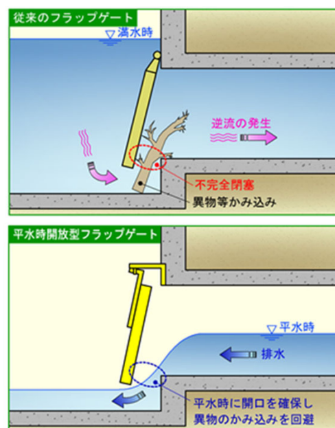
図1 従来のフラップゲートと平水時開放型フラップゲートの比較
