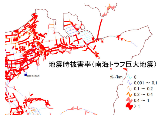
図4 管路被害予測結果の図面化
