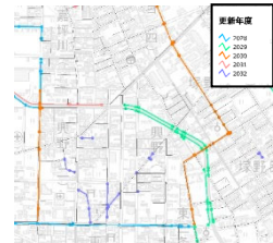
図10 更新・耐震化年次計画図面のイメージ
