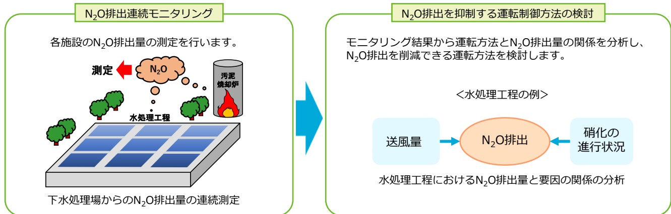
図5 N 2 O生成抑制調査
