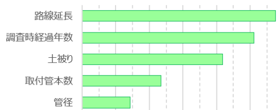
劣化予測に寄与の大きいパラメーターの抽出例
