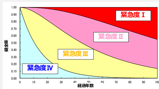
従来の健全率予測
